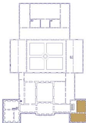
Planta 8 – Terceiro pavimento – Biblioteca Particular de Sua Majestade Imperial
